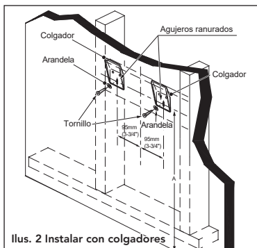
Ilus. 2 Instalar con colgadores
